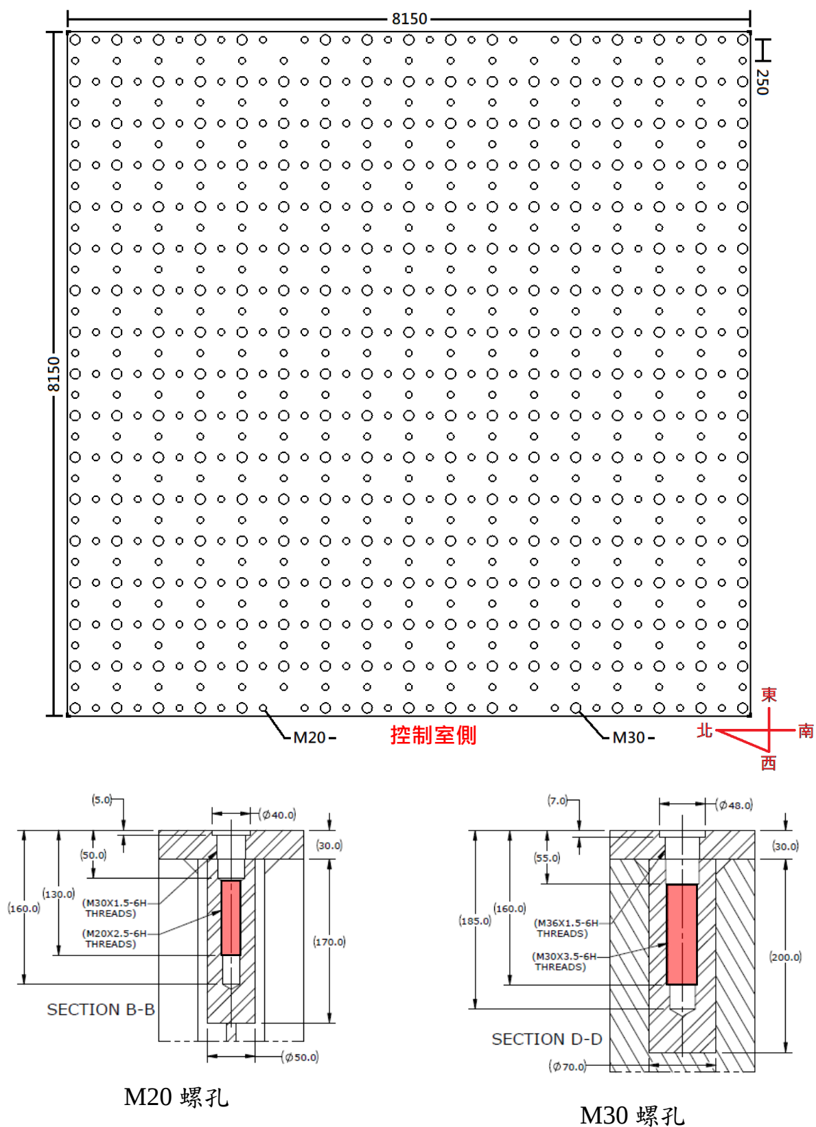
圖2.4 振動台螺孔分布及洞徑規格 (單位：mm)
