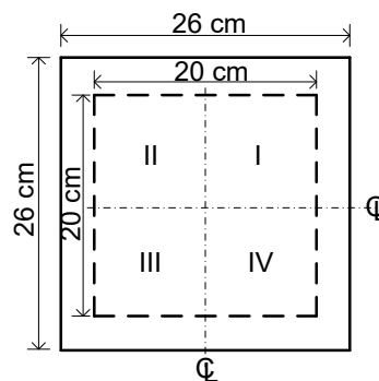
圖 2 模型建置範圍
