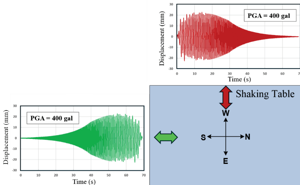
圖 6 輸入之位移歷時及方向
