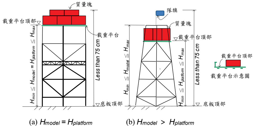
圖 3 模型立面示意圖
