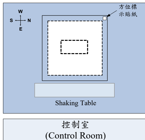
圖 4 模型於振動台之安裝方向示意圖
