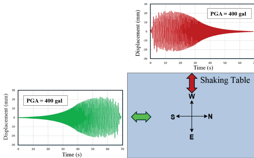
圖 6 輸入之位移歷時及方向
