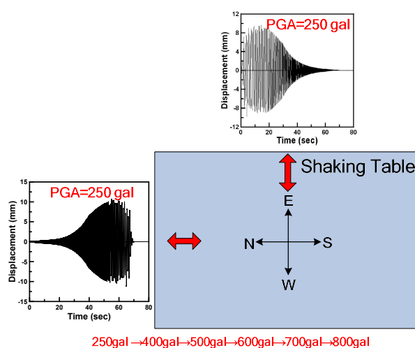
圖 5 輸入之位移歷時及方向
