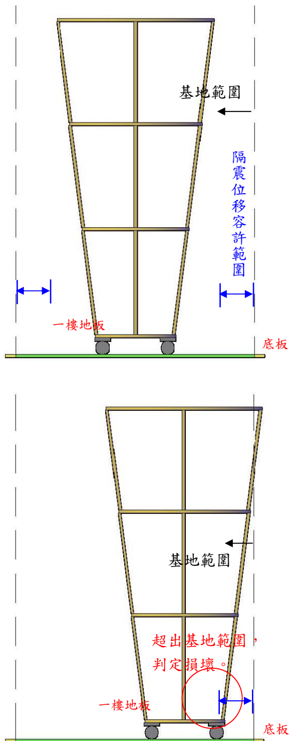
圖 5 隔震系統位移容許範圍示意圖
