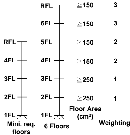
圖 3 模型樓層定義、樓地板面積要求及鐵塊權重說明
