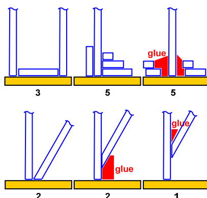
圖 3 底板木條數計算例
