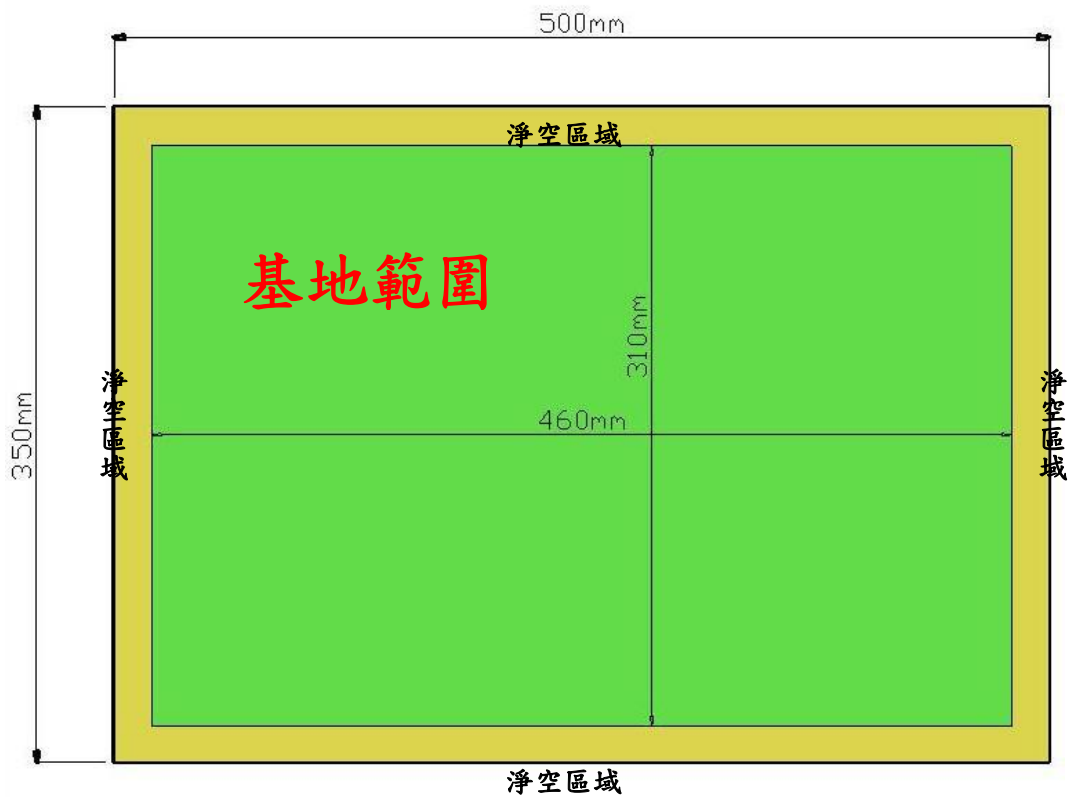
圖 2 木質密集版底座俯視圖
