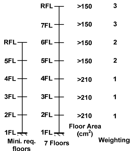
圖 4 模型樓層定義、樓地板面積要求及鐵塊權重說明
