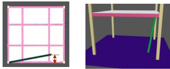
圖 13 模型內外斜撐說明
