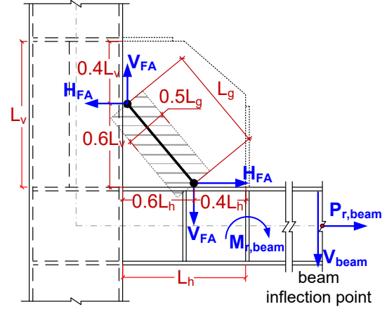
圖 5 隅板等效支撐模型
