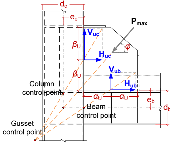
圖 4 泛均力法隅板之力量分布
