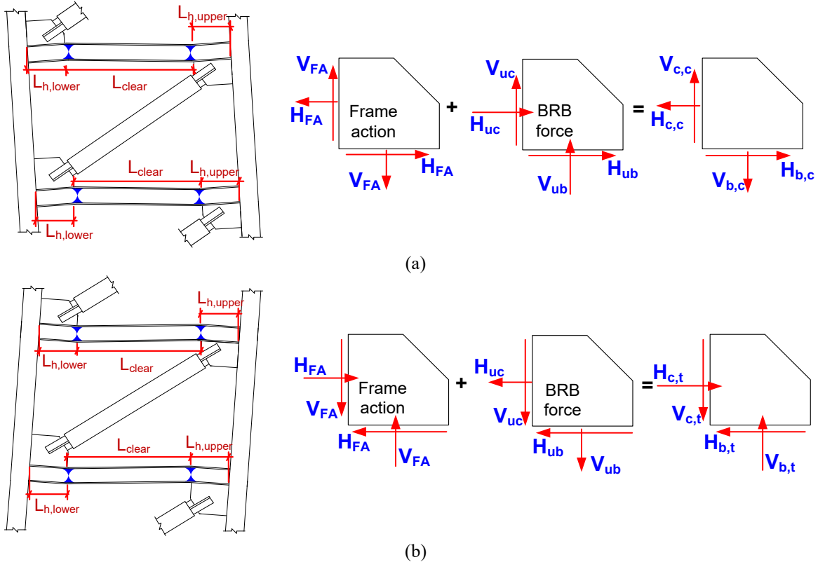
圖 6 梁柱角隅隔板受斜撐軸力與梁柱開合效應受力情形(a) 斜撐受壓梁柱接合處張開，與(b)斜撐受拉時梁柱接合處閉合
