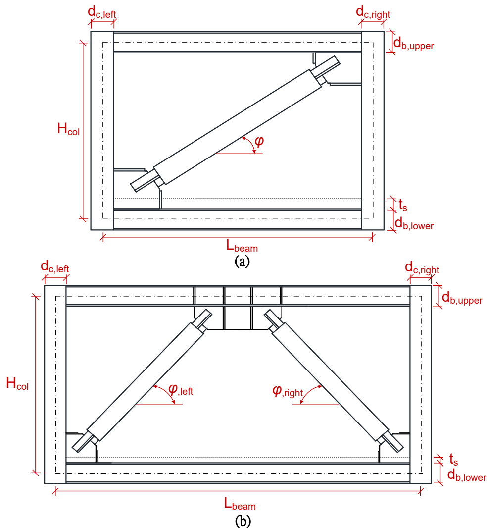
圖 1 (a)單斜與(b)雙斜配置槽接式挫屈束制支撐構架尺寸示意圖
