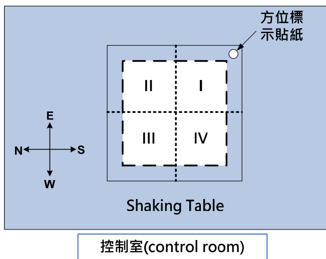
圖 3 模型於振動台之安裝方向示意圖
