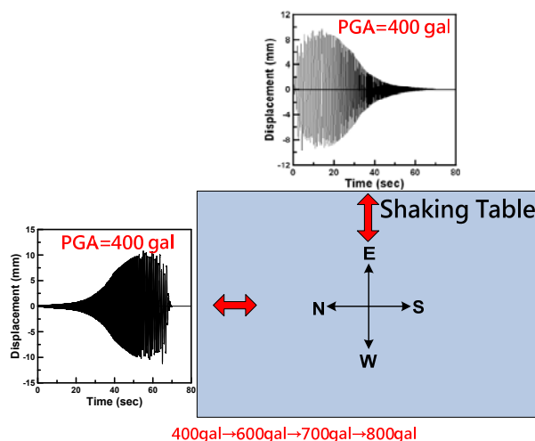
圖 5 輸入之位移歷時及方向
