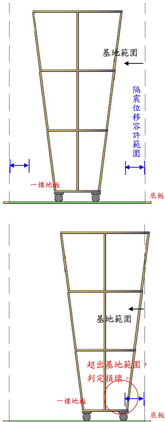
圖 5 隔震系統位移容許範圍示意圖
