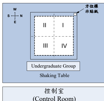
圖 3 模型於振動台之安裝方向示意圖
