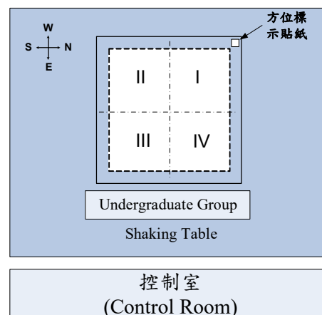
圖 3 模型於振動台之安裝方向示意圖
