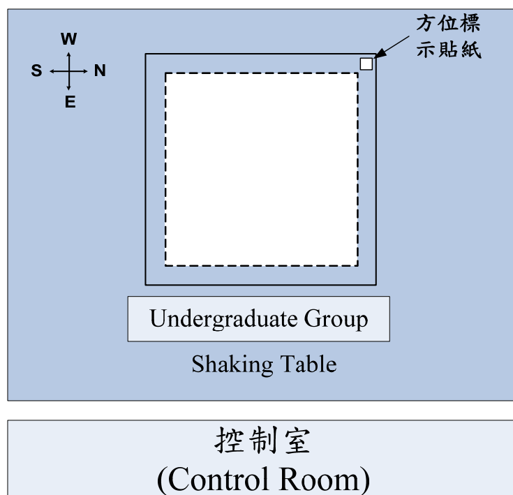
圖 12 模型於振動台之安裝方向示意圖
