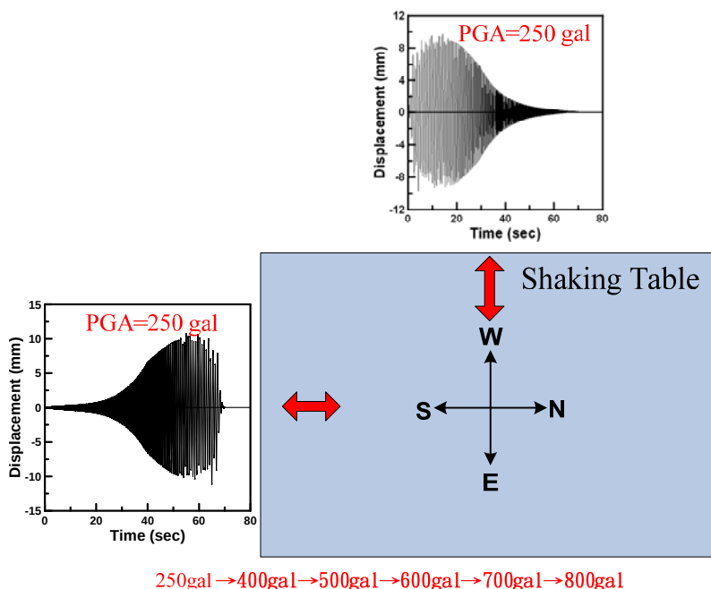
圖 15 輸入之位移歷時及方向
