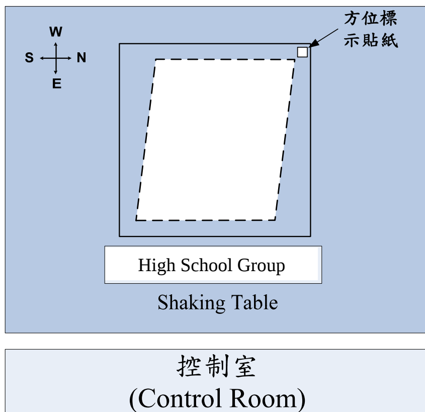
圖 13 模型於振動台之安裝方向示意圖
