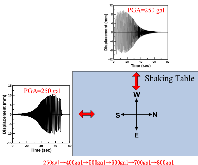
圖 15 輸入之位移歷時及方向
