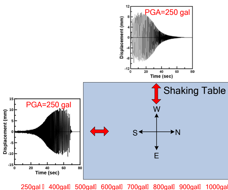
圖 14 輸入之位移歷時及方向
