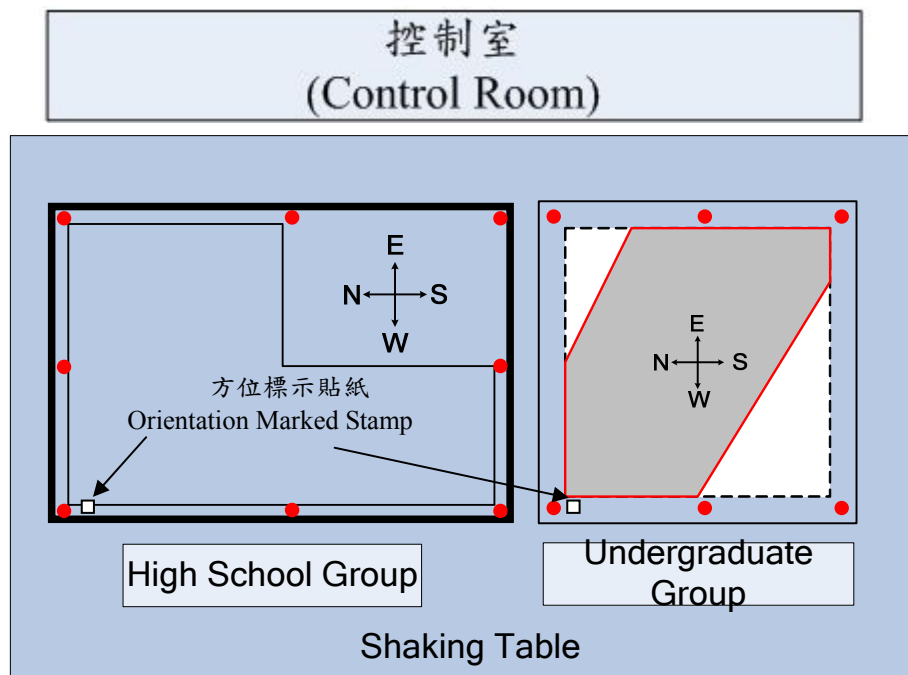
圖 14 模型於振動台之安裝方向示意圖
