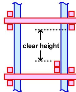
圖 6 樓層淨高示意圖
