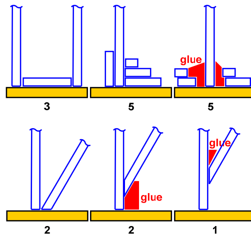
圖 3 底板木條數計算例
