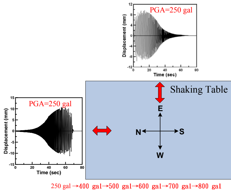
圖 12 輸入之位移歷時及方向
