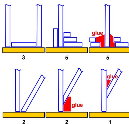
圖 3 底板木條數計算例
